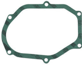
CÓD. 20.410 JC DESC. JUNTA DA CAIXA À CARÇAÇA DE EMBREAGEM MAT. NA N.ORIG.
