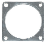
CÓD. 150.623 CH DESC. JUNTA DO COLETOR DE ESCAPAMENTO MAT. CH N.ORIG.
