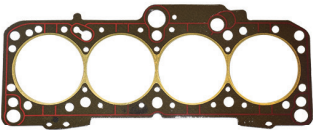
CÓD. 30.601 GAS DESC. JUNTA DO CABEÇOTE MAT. BBS N.ORIG.
